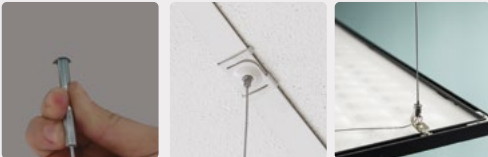
FIXATIONS PLAFOND Dalle béton - plaque de plâtre - ossature T24 - plafond bois
